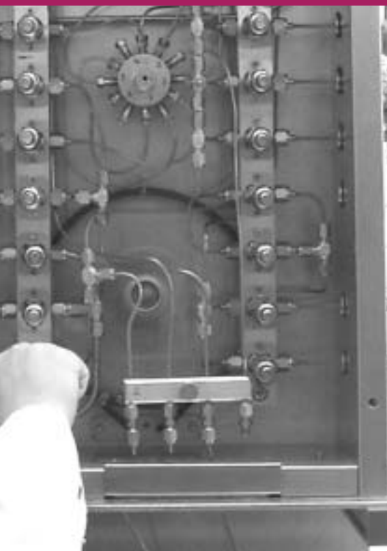
Membranreaktor im Betrieb
