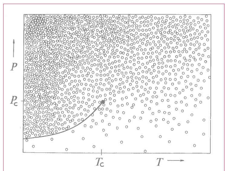
Druck und Temperatur beeinflussen die Dichte des Kohlendioxids.
