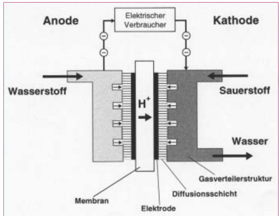
Funktionsprinzip einer Brennstoffzelle mit Austauschmembran für Protonen ( H^+ )
