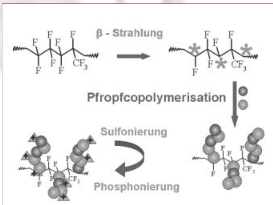
Schematische Herstellung der neuartigen Protonenaustauschmembran
