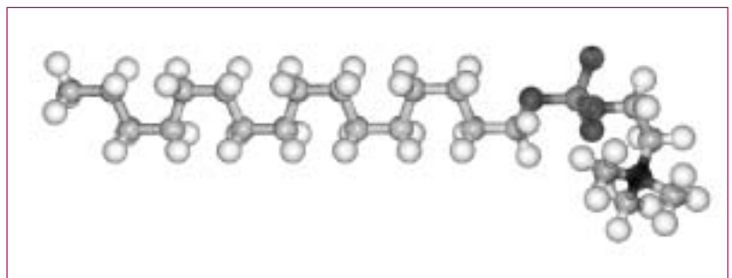
Hexadecylphosphocholin – gesättigte Alkylkette mit 16 Kohlenstoffatomen
