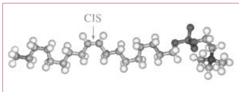
Oleylphosphocholin – ungesättigte Alkylkette mit 18 Kohlenstoffatomen und cis-Doppelbindung
