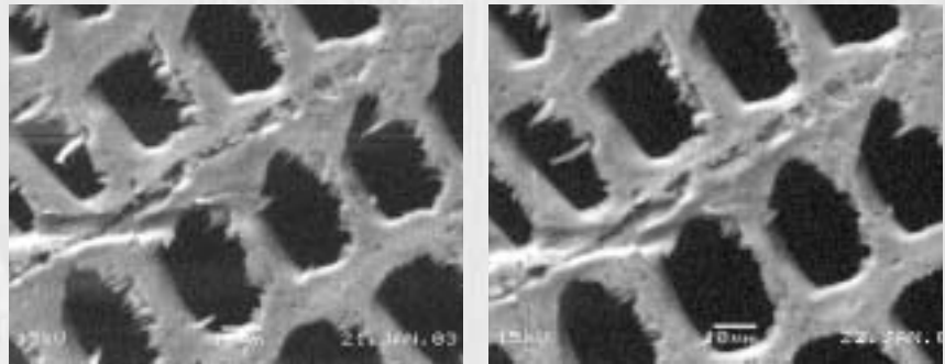
Fichtenholz vor (links) und nach der Plasmabehandlung (Aufnahme im Rasterelektronenmikroskop)
