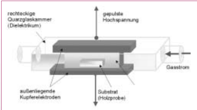
Schema einer Barriereentladungsapparatur
