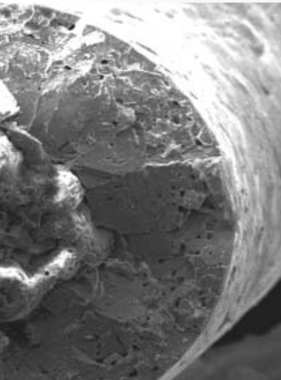
icid überzogen (Querschnitt im Rasterelektronen-Titan gänzlich zu Titansilicid reagieren.
