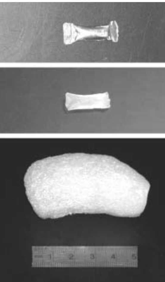
Probenkapsel, wasserhaltiges Glas und durch Erhitzen gewonnener künstlicher Bimsstein
