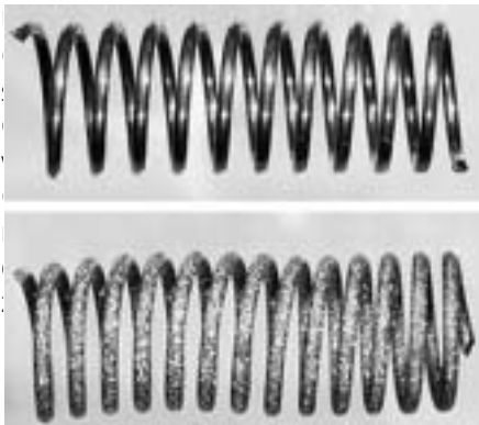
Aus dem Eisendraht hat sich nach der Behandlung Eisensilicid gebildet, die Spiralform blieb dabei erhalten.
