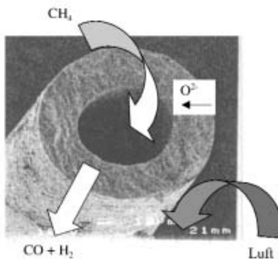
Membranunterstützte Partialoxidation von Erdgas zu Synthesegas an einer Perowskithohlfaser (Faserproduktion am FHI für Grenzflächen- und Bioverfahrenstechnik Stuttgart): Durch Sauerstoffionendiffusion gelangt Sauerstoff aus der Umgebungsluft in das Innere der Kapillare, wo die Reaktion des Methans zum Synthesegas erfolgt.
