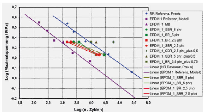
Wöhlerlinien von EPDM- Dienkautschukverschnitten im Vergleich zu einem herkömmlichen EPDM-Werkstoff und einem NR-Praxiswerkstoff
